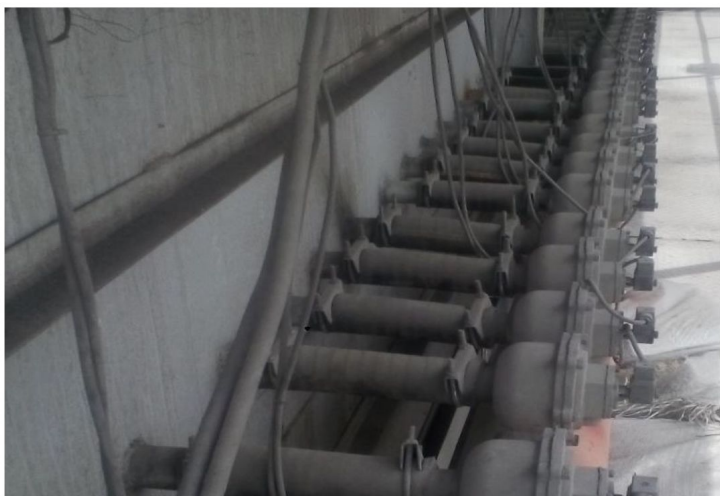
اجرای جت فیلتر و اتوماسیون فیلترینگ
